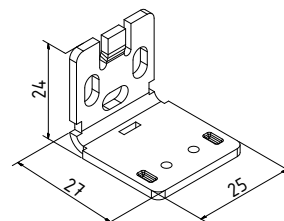
MONTÁŽNÍ KONZOLA
