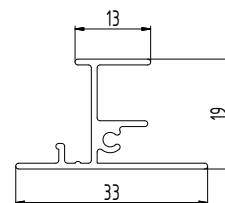
VODICÍ LIŠTA
